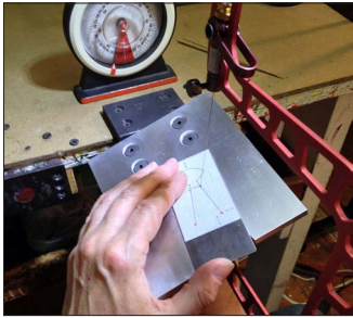
Sawing a Blanking Die
